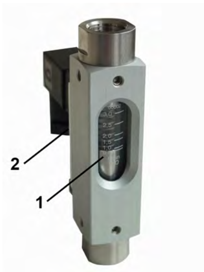
Abb. 1: Strömungswächter RVO/U-4
