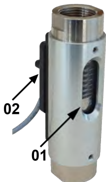
Abb. 1: Strömungswächter DKG-1
