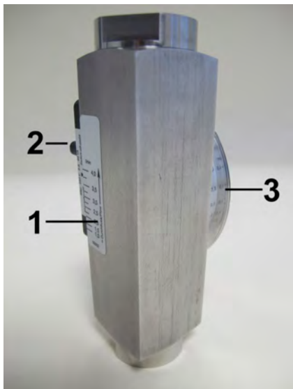
Abb. 1: Strömungswächter DKME/A-1
