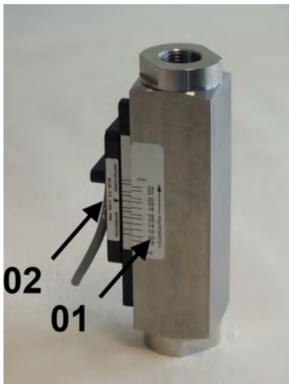
Abb. 1: Strömungswächter DKME-1
