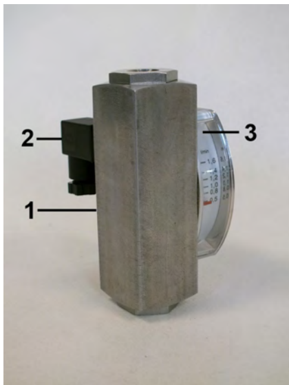
Abb. 1: Strömungswächter DKM/A-2
