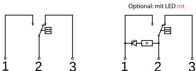
Abb. 3: Anschlussbilder
